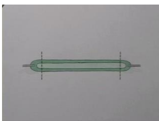
⑥冷めると中空の管ガラスが完成
